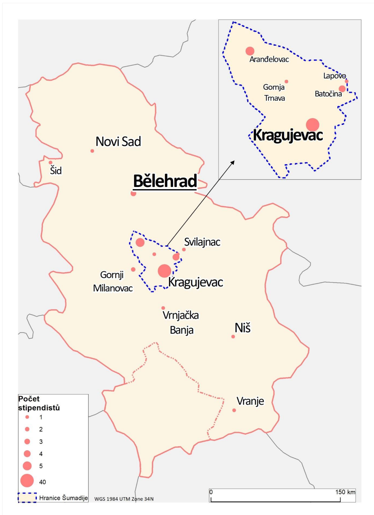
Obr. 3 Místo pobytu před příjezdem do Jihomoravského kraje Zdroj: MapCruzin, 2018; Geofabrik, 2018; Natural Earth data, 2018
